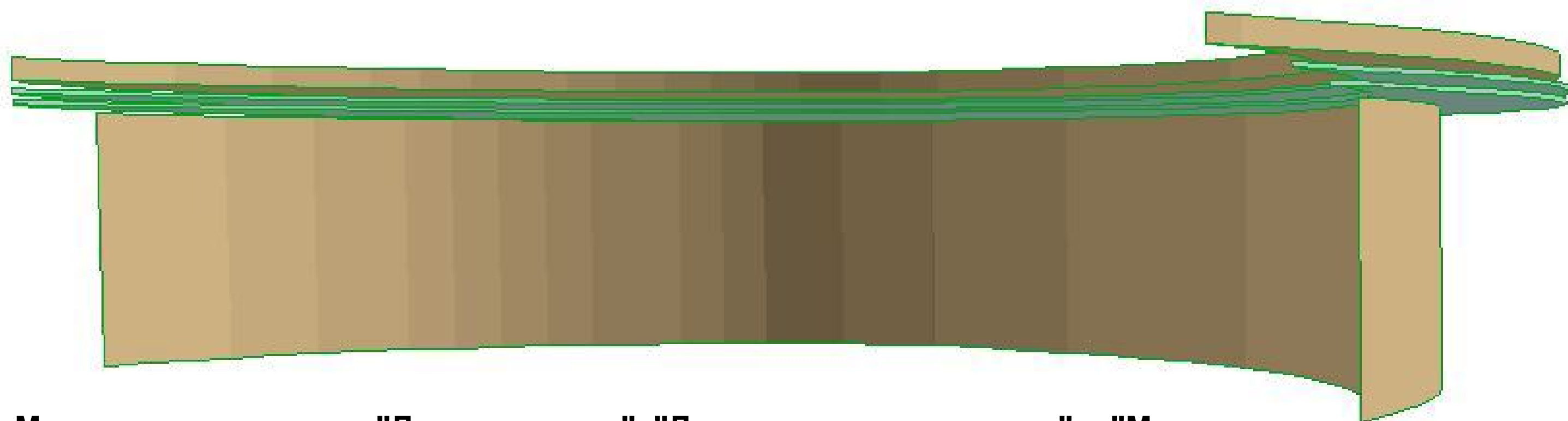
Маса за предаванията "Денят започва", "Денят започва с култура" и "Малки истории" Изработва се от желязни профили с огъвки и МДФ боядисан с полиоританова боя. Между плота и основата се монтират зелени плексигласови плочи със заоблена форма. Дебелината на плексигласа е 7мм.
