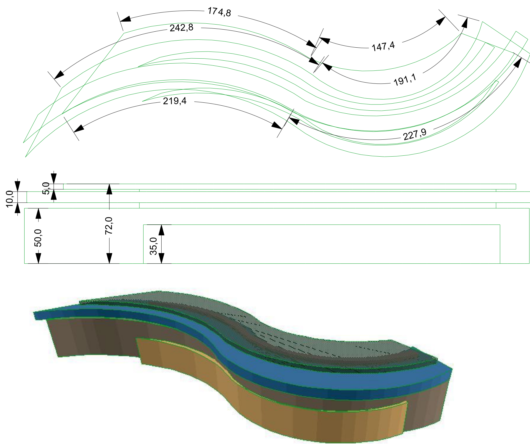
Бюро за "Кът за четене на новини" Изработва се от желязни профили с огъвки покрити с МДФ боядисан с полиоританова боя.
