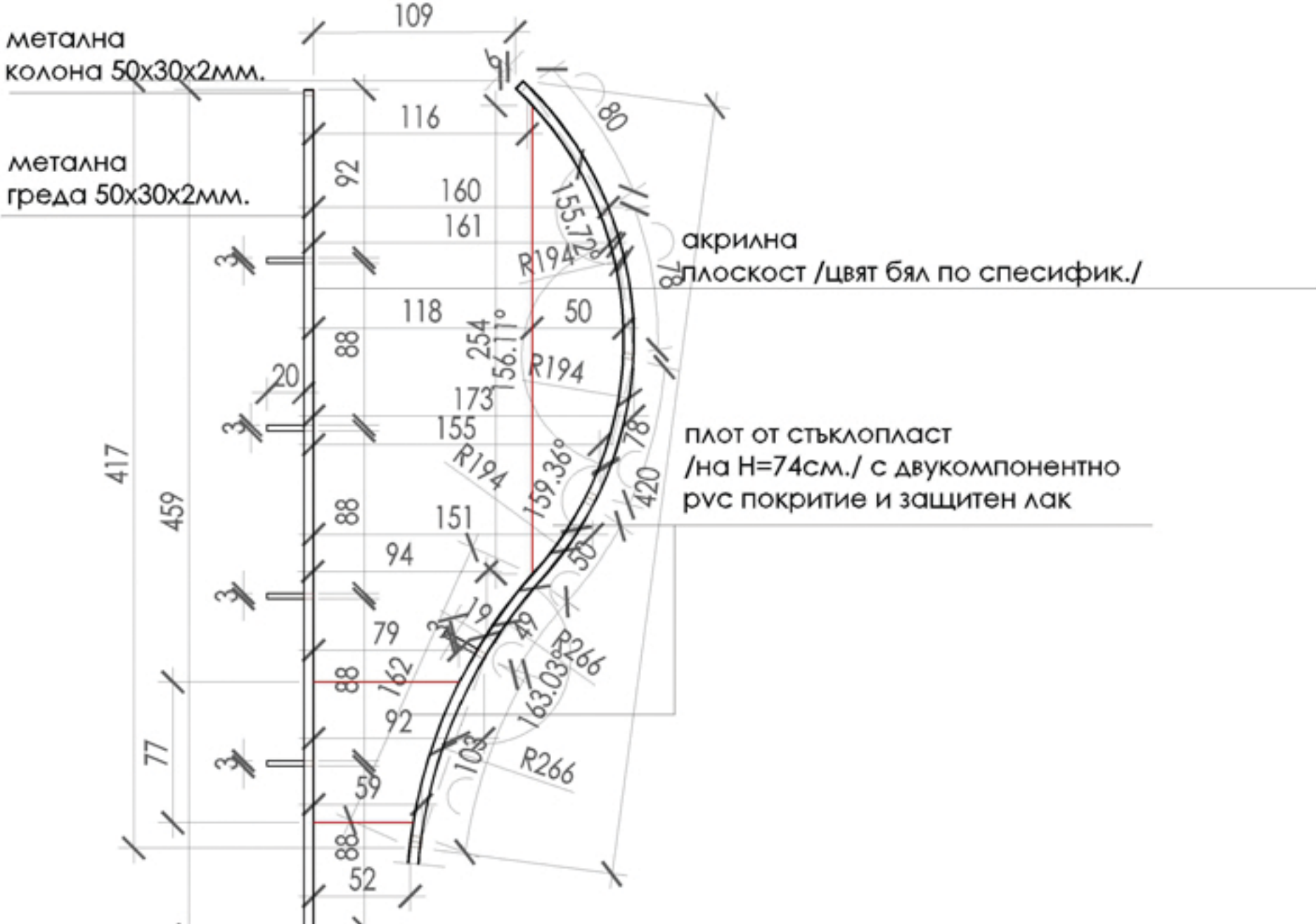
ДЕТАЙЛ III - КЪТ ЗА ЧЕТЕНЕ НА НОВИНИ
