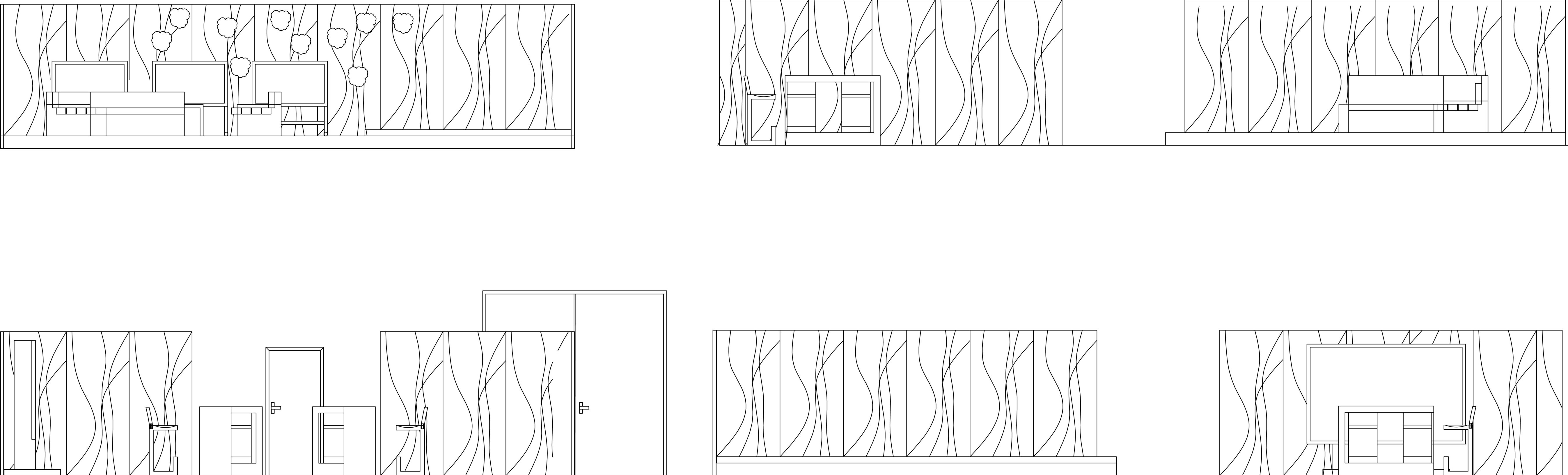
Разрези 1:20
