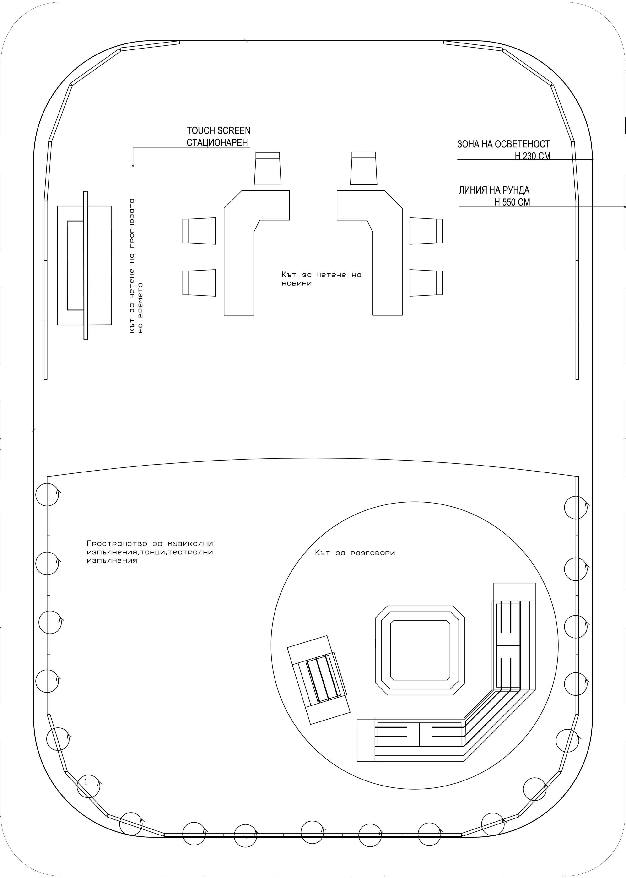
План кътове 1:20
