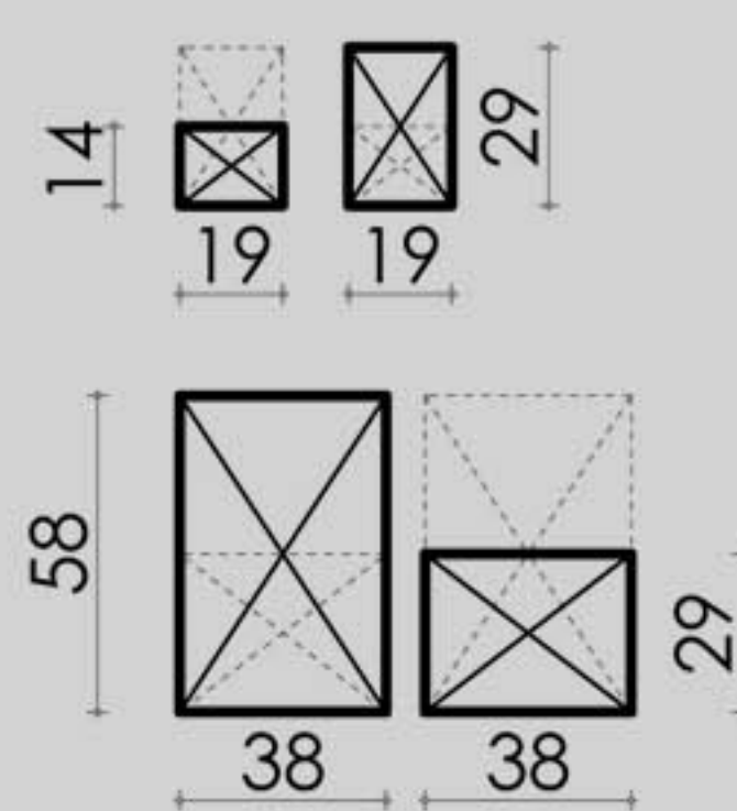
РАСТЕР - ПРЕГРАДНА МРЕЖА
